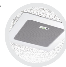
BEAMFORMING ATND1061 MICROFONE PROFISSIONAL DE TETO PERMITE DEFINIR 32 ZONAS DE CAPTAÇÃO ENTRADA E SAÍDA DE ÁUDIO ANALÓGICO DSP E CANCELAMENTO DE ECO ACÚSTICO (AEC)
