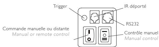
Panneau de contrôle Control panel
