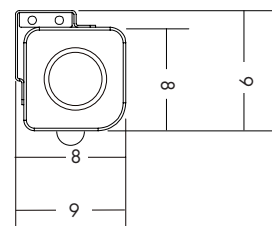
Côté du carter avec patte de fixation Side of the case with bracket
