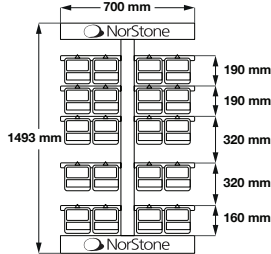
COMBINAISON 1 Packs câbles uniquement Cables packs only
