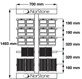
COMBINAISON 2 Packs et rouleaux de câbles Cables packs and rolls assembly
